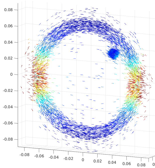
Figura 2.3: Distribución del campo eléctrico en una sección del eje y , dado por la inyección de corriente entre los electrodos T7 y T8 de la figura 2.2. Los vectores en rojo son los de mayor intensidad, y en azul los de menor intensidad. La diferencia entre la cantidad de flechas en cada zona, corresponde a que el mallado en esa zona tiene una resolución mayor o menor, según el caso.
