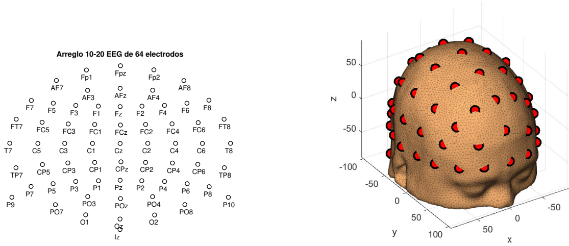
Figura 3.5: Arreglo 10-20 de 64 electrodos. A la izquierda, una proyección del arreglo en el plano. A la derecha, vista superior-derecha del arreglo colocado en el modelo realista.
